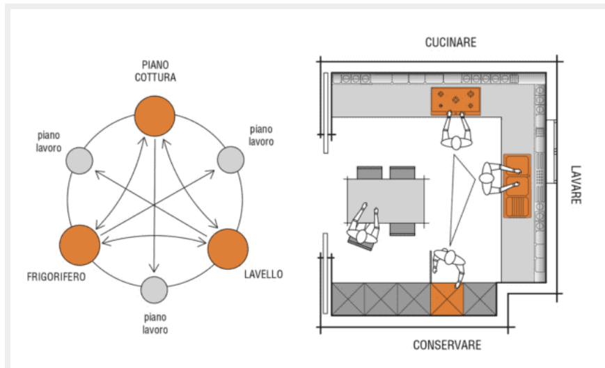
Pianta di una cucina a U con indicato il "triangolo di lavoro" ideale. Tratto da www.valcucine.it
